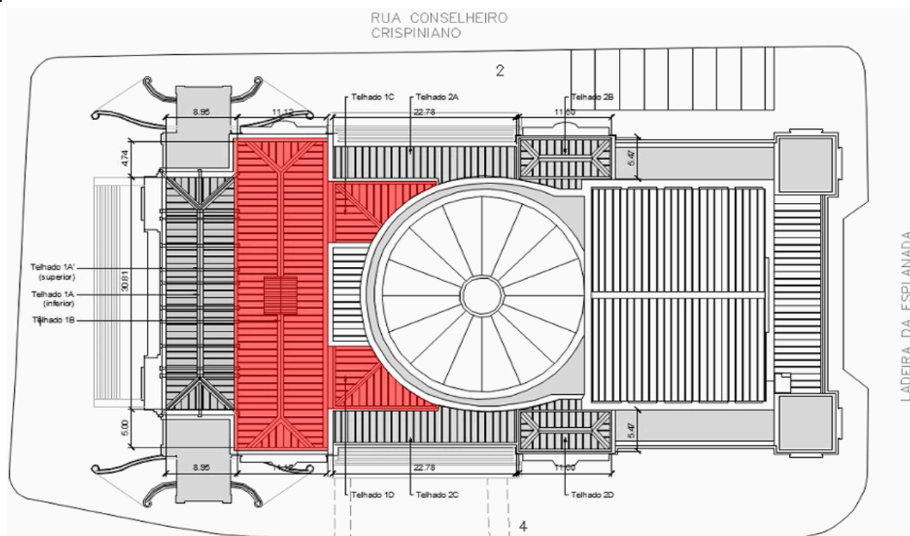
Fig. 01 - Planta de cobertura do Teatro Municipal de São Paulo com demarcação em vermelho do telhado 1B, 1C e 1D
