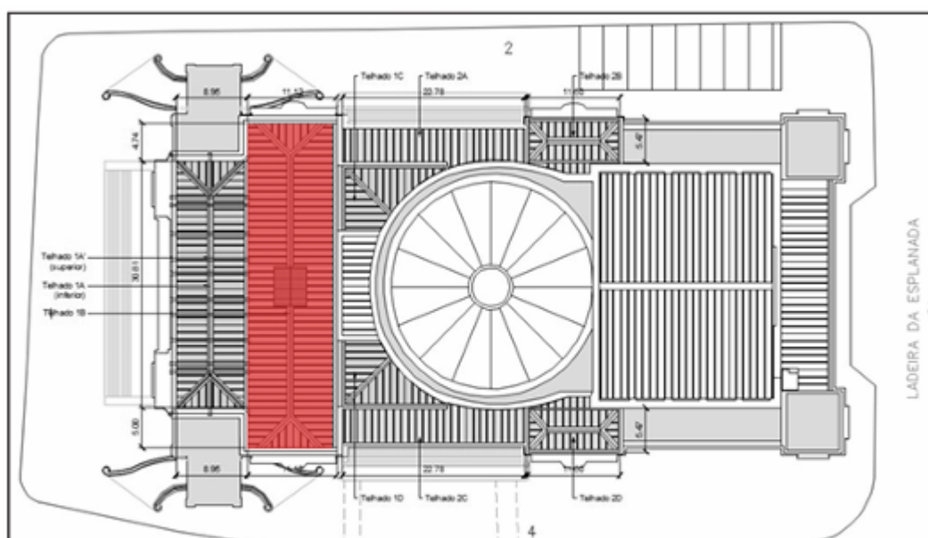
Fig. 01 - Planta de cobertura do Theatro Municipal de São Paulo com demarcação em vermelho do telhado 1B
