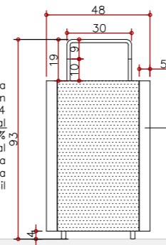
VISTA FRONTAL ESC 1:25
