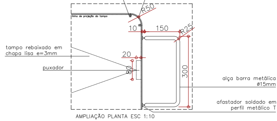
AMPLIAÇÃO PLANTA ESC 1:10
