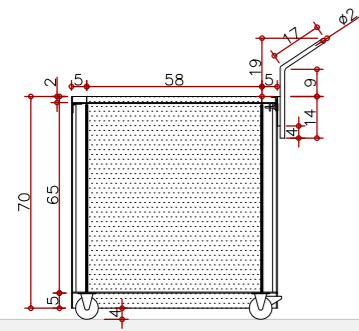
VISTA LATERAL ESC 1:25
