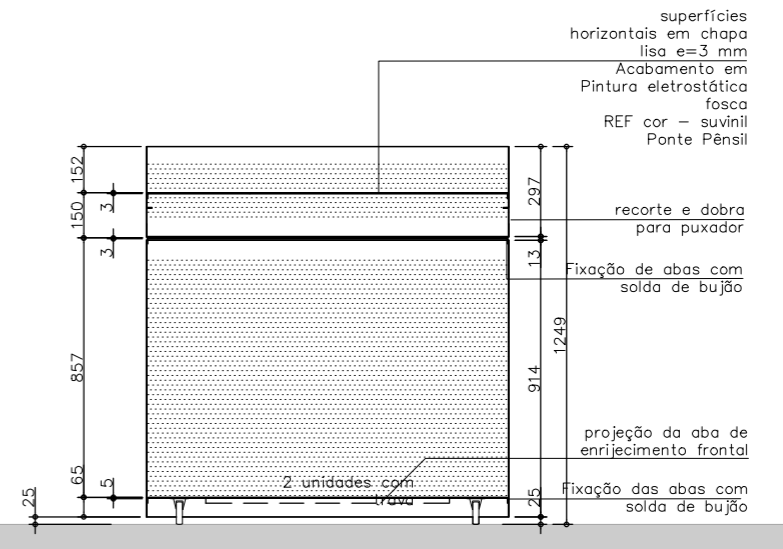
CORTE LONGITUDINAL ESCALA 1:25
