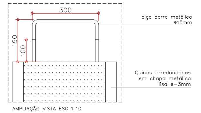
AMPLIAÇÃO VISTA ESC 1:10
