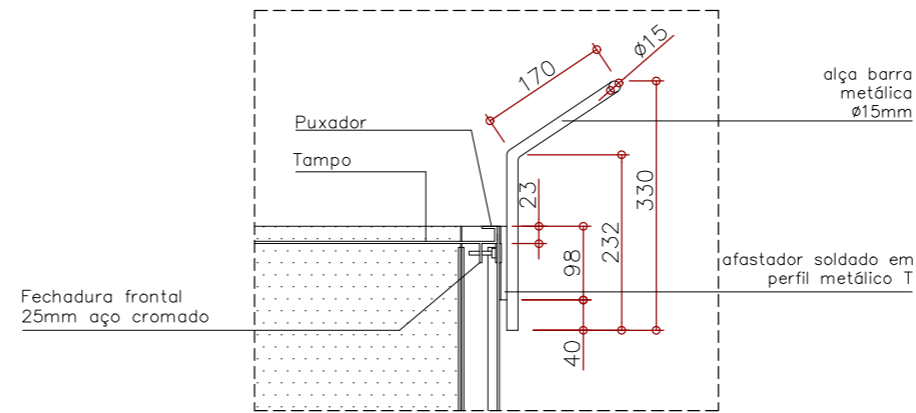
AMPLIAÇÃO CORTE LONGITUDINAL ESC 1:10
