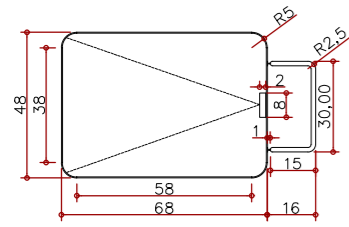
PLANTA ESC 1:25
