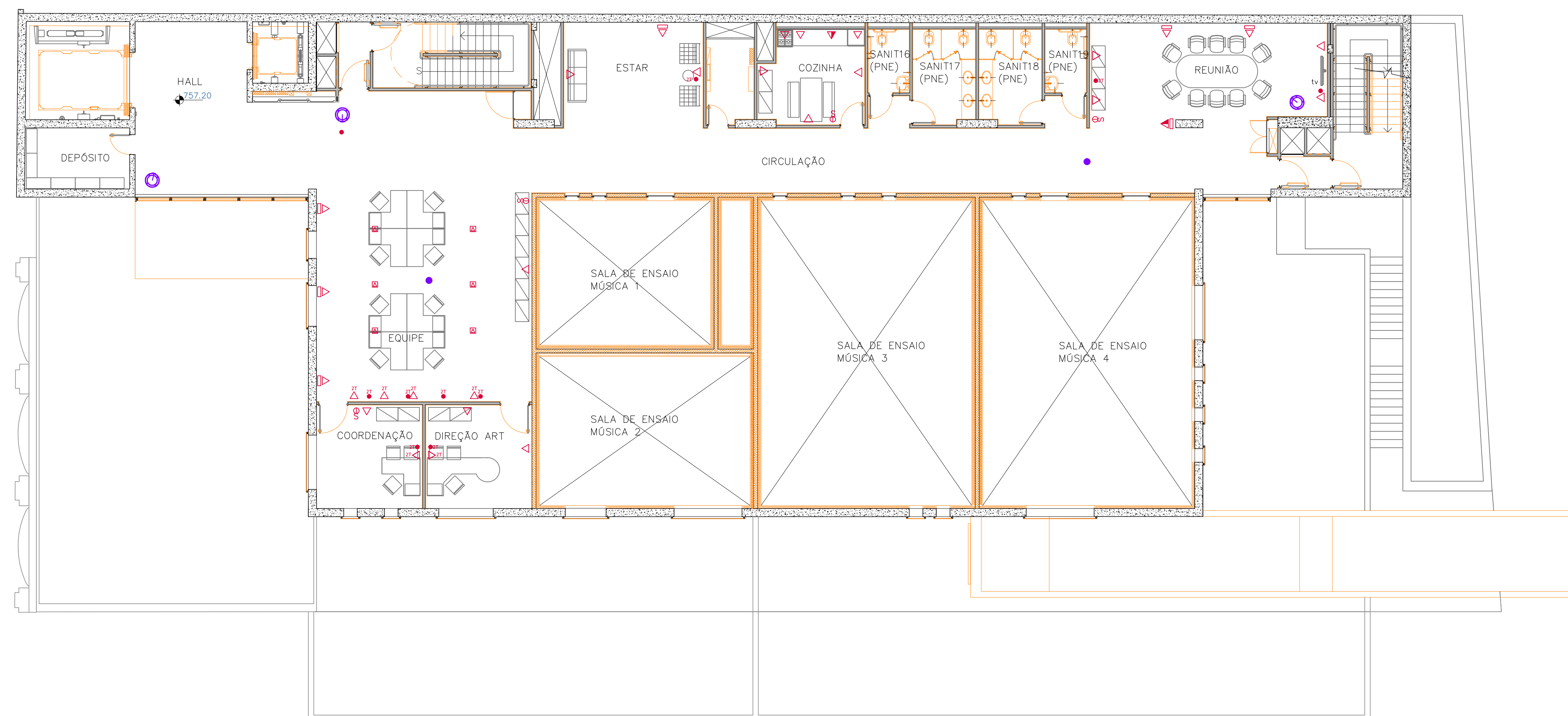
EDIFÍCIO CORPOS ARTÍSTICOS PRAÇA DAS ARTES PLANTA LAYOUT 6º PAVIMENTO - ESCALA 1:100
