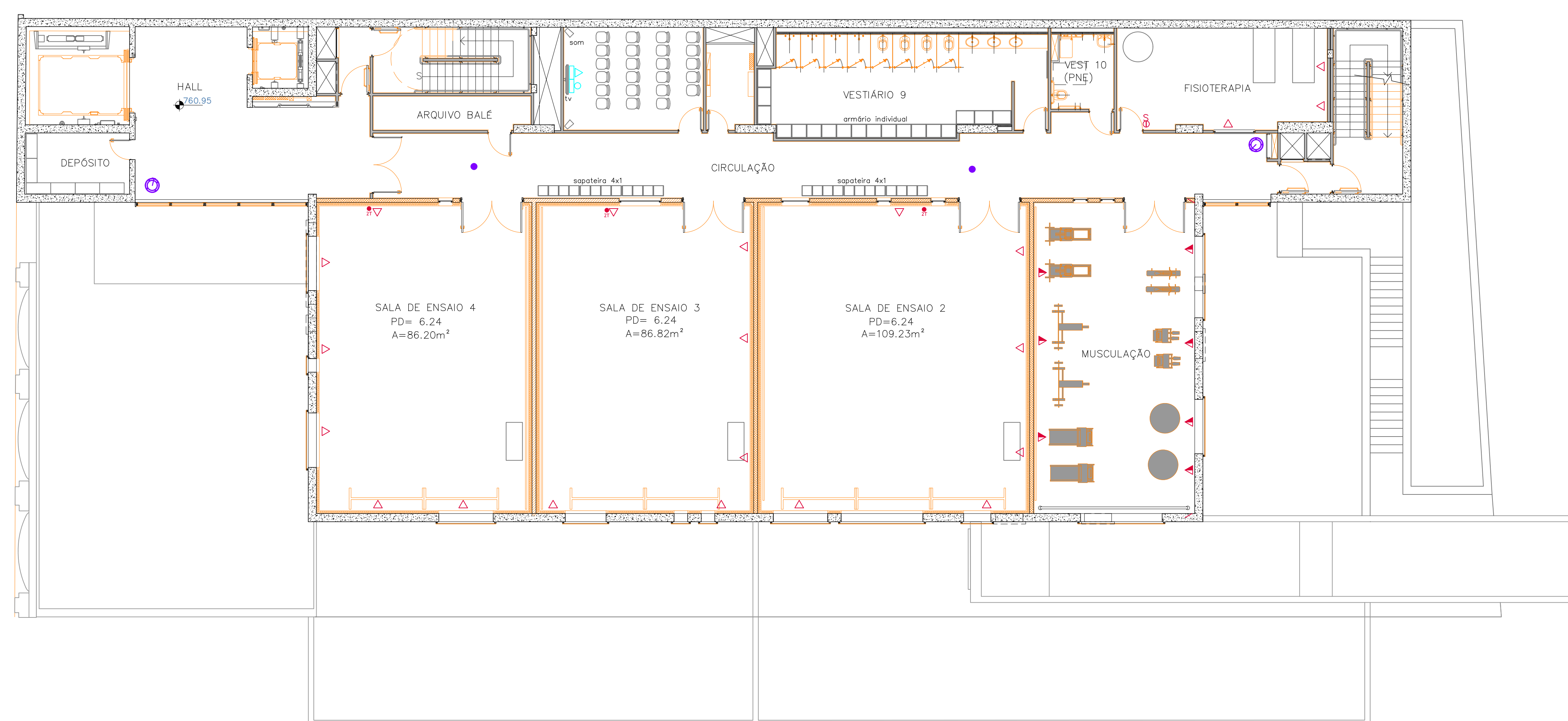
EDIFÍCIO CORPOS ARTÍSTICOS PRAÇA DAS ARTES PLANTA LAYOUT 7º PAVIMENTO - ESCALA 1:100
