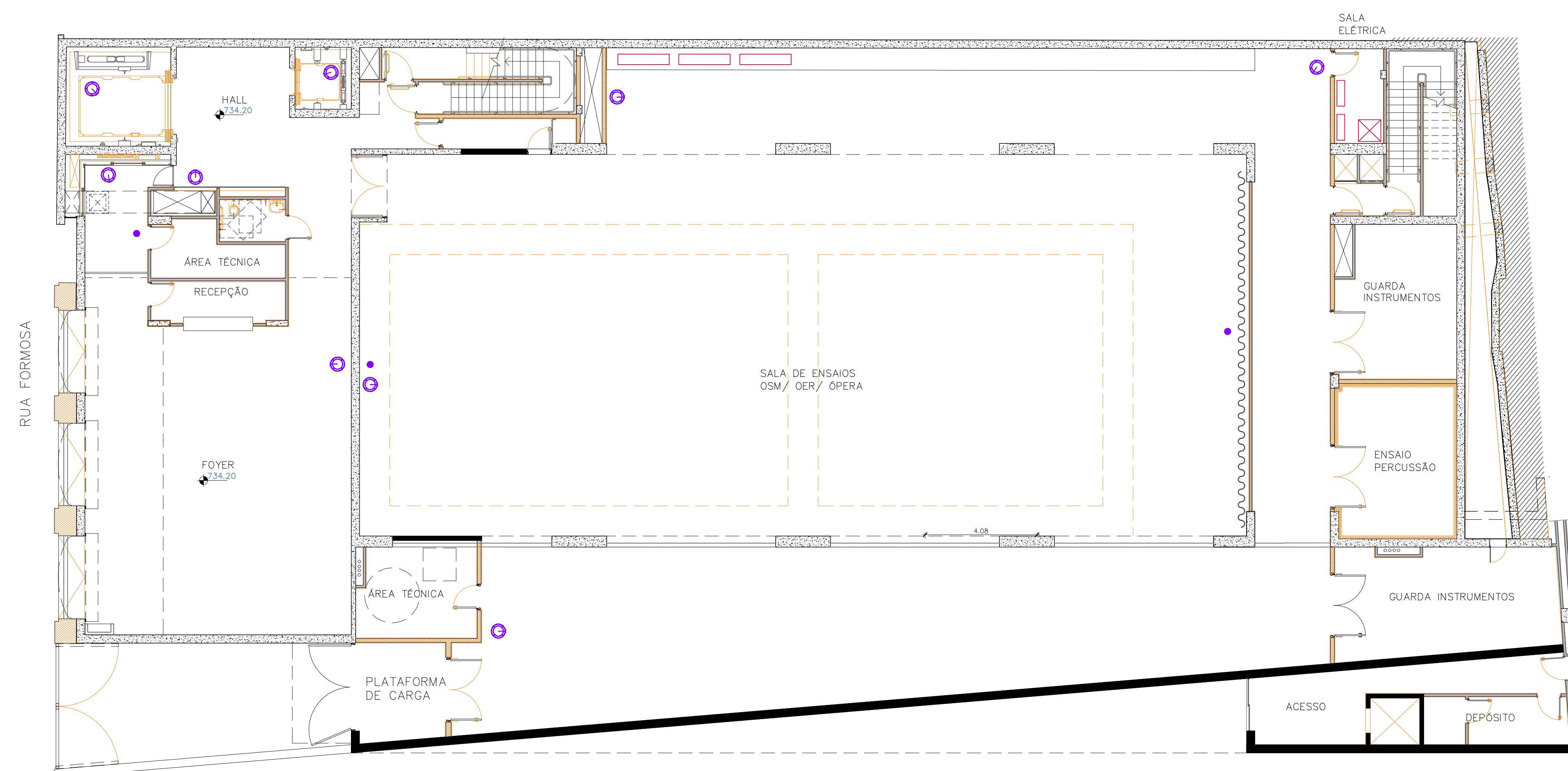
EDIFÍCIO CORPOS ARTÍSTICOS PRAÇA DAS ARTES PLANTA LAYOUT - TÉRREO NÍVEL 734,20 - ESCALA 1:100
