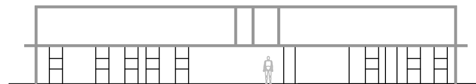
BLOCO 5 - CORTE BB' ESC. 1:250
