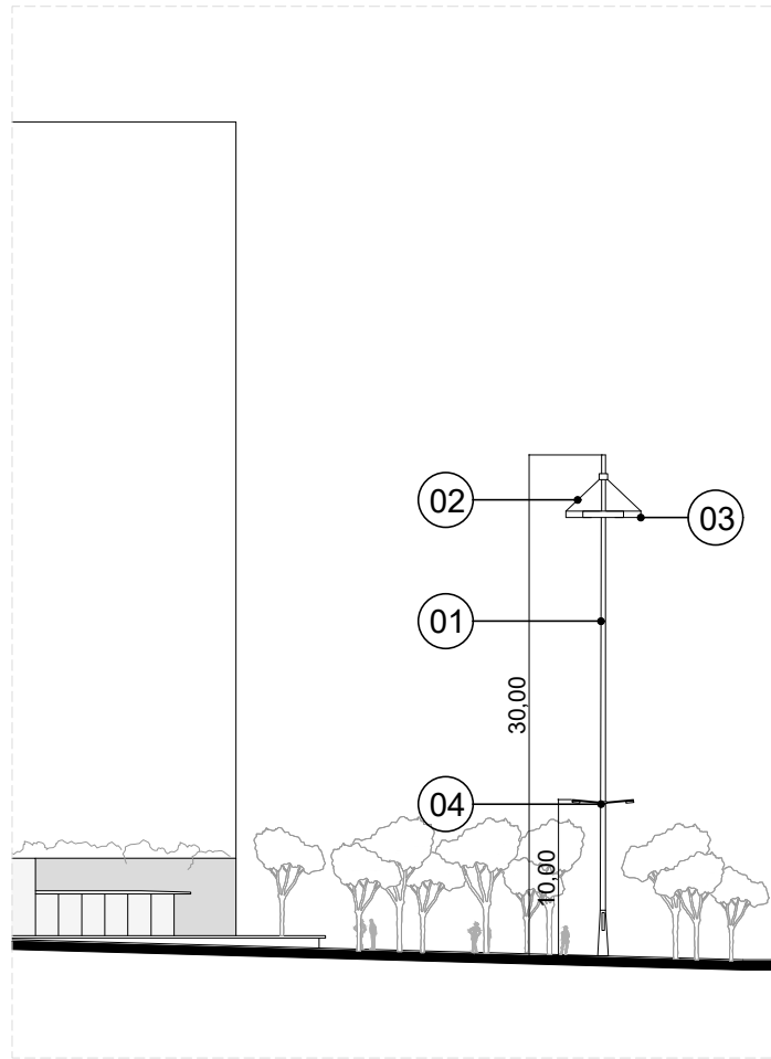
SITUAÇÃO PROPOSTA ESC. 1:500
