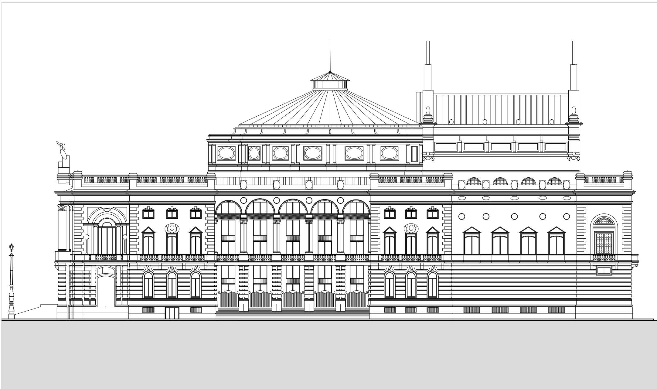
TMSP - THEATRO MUNICIPAL DE SÃO PAULO ELEVAÇÃO CORONEL XAVIER DE TOLEDO ESC. 1:350
