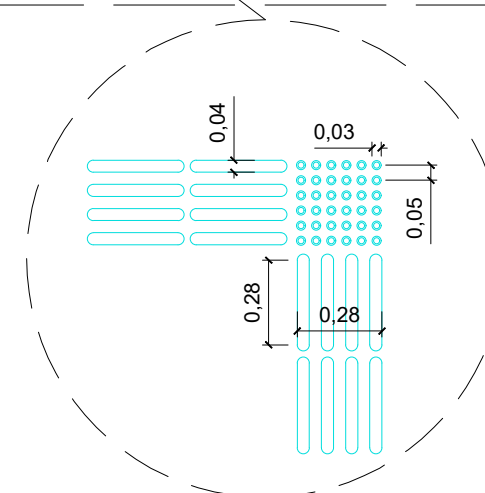
EXEMPLIFICAÇÃO DE PISO TÁTIL SITUAÇÃO S/ ESCALA
