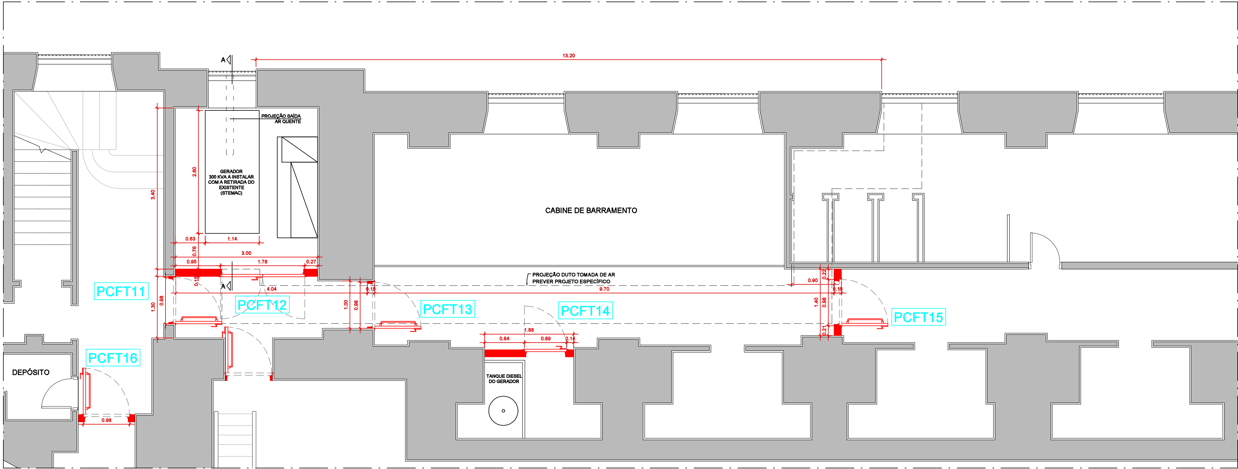
PLANTA - PAVIMENTO TÉRREO SALA DO GERADOR EBC. 150
