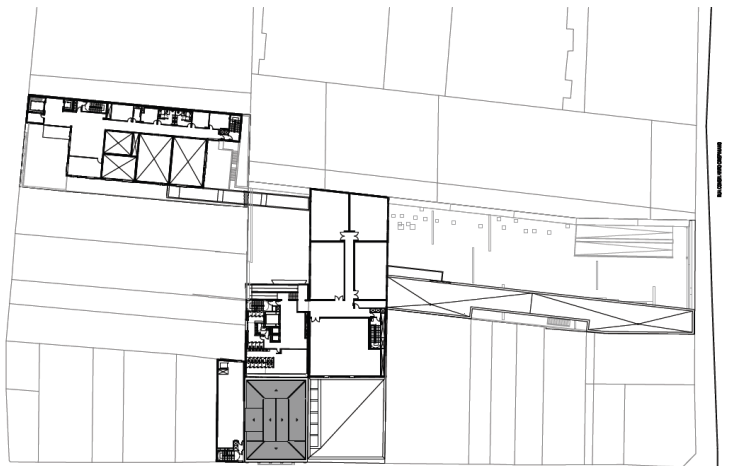
5º pavimento
