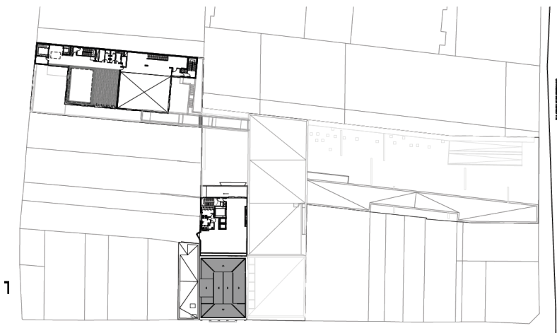
9º pavimento
