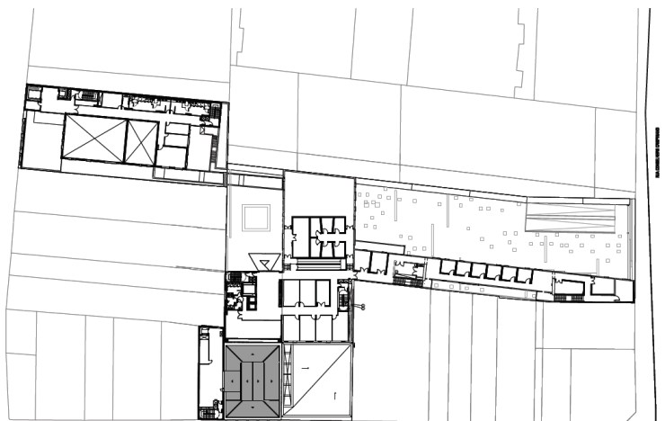
3º pavimento
